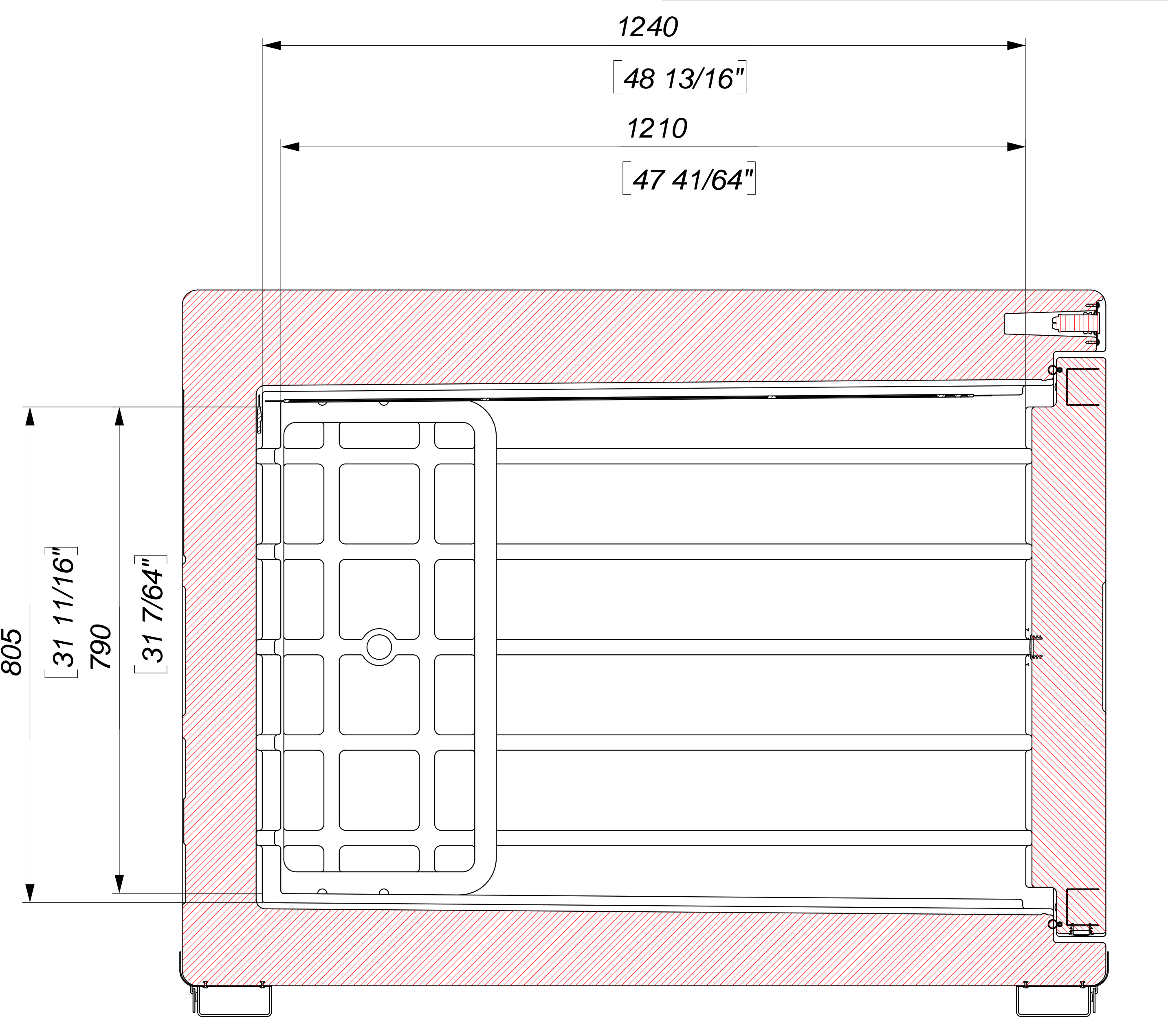
Sezione E-E SCALE 1 : 5
