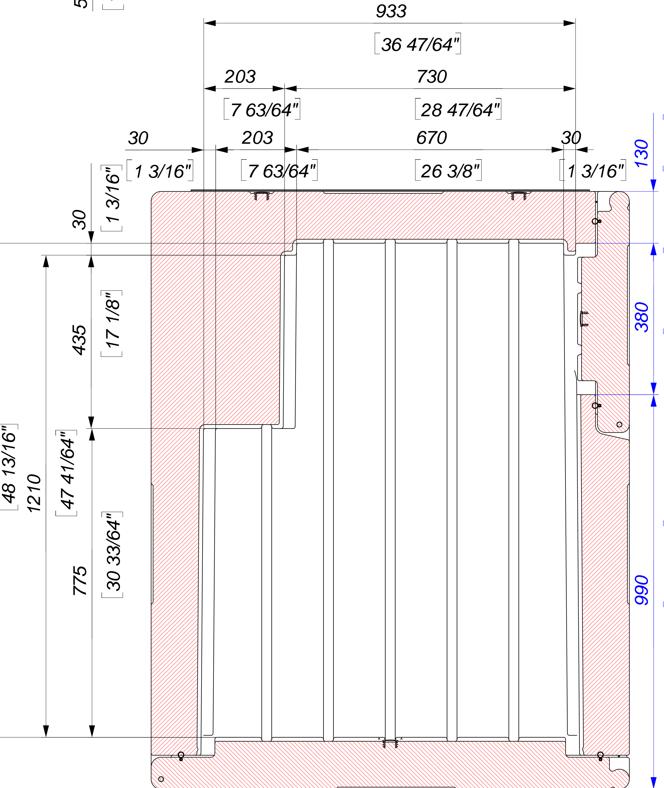
Sezione F-F SCALE 1 : 5
