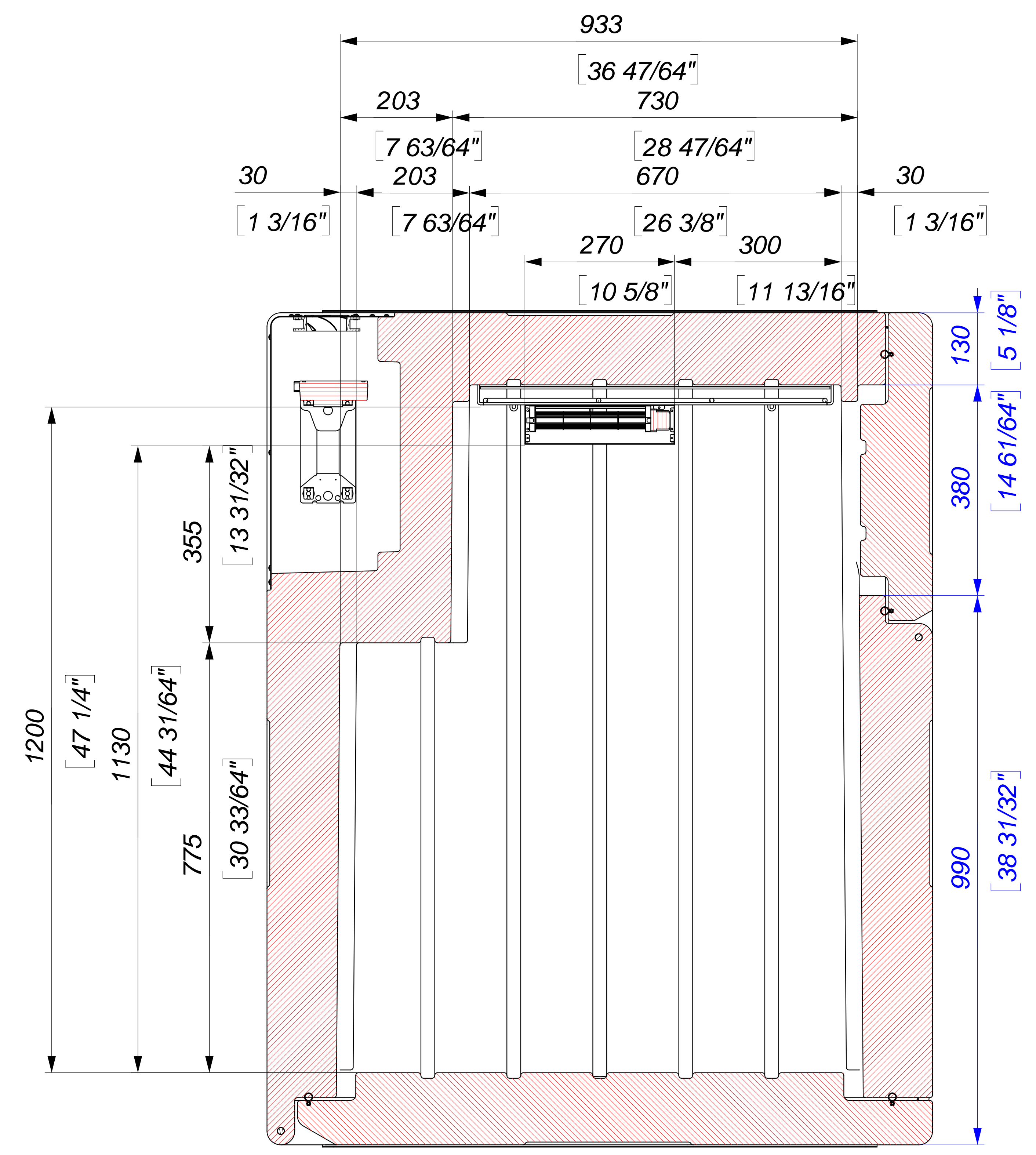
Sezione F-F SCALE 1:5
